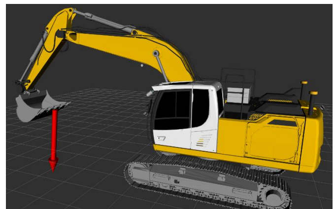
Abbildung 1: Autonome Bagger mit Hydraulikdrucksensoren und geschätzte Kraft am Endeffektor
